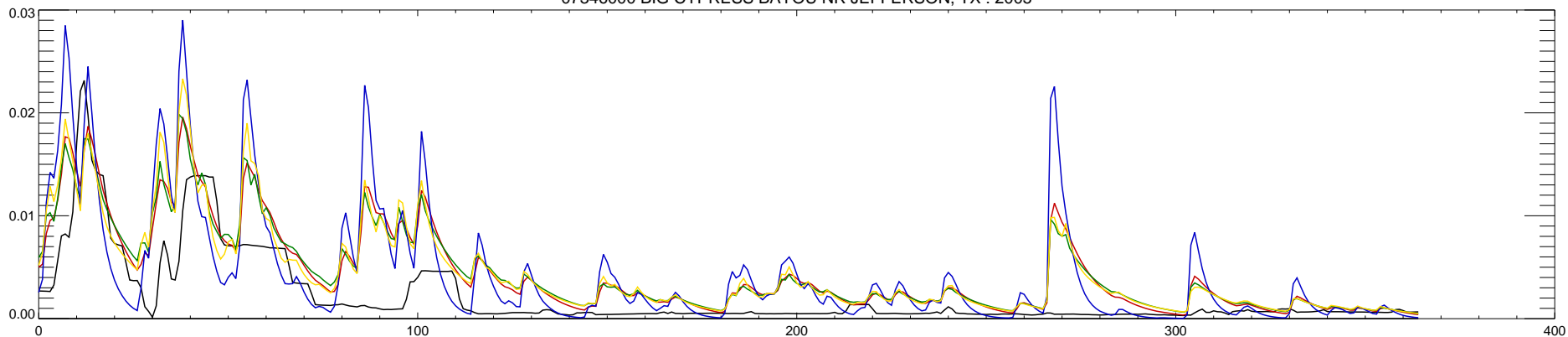
07346000 BIG CYPRESS BAYOU NR JEFFERSON, TX : 2006
