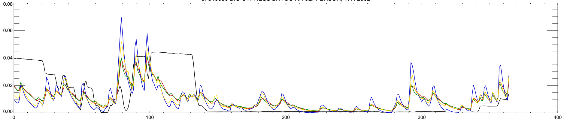
07346000 BIG CYPRESS BAYOU NR JEFFERSON, TX : 2003
