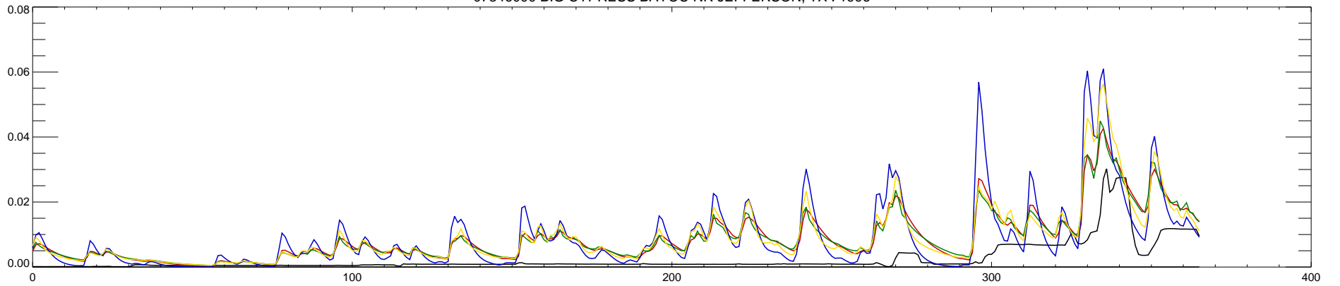
07346000 BIG CYPRESS BAYOU NR JEFFERSON, TX : 1997
