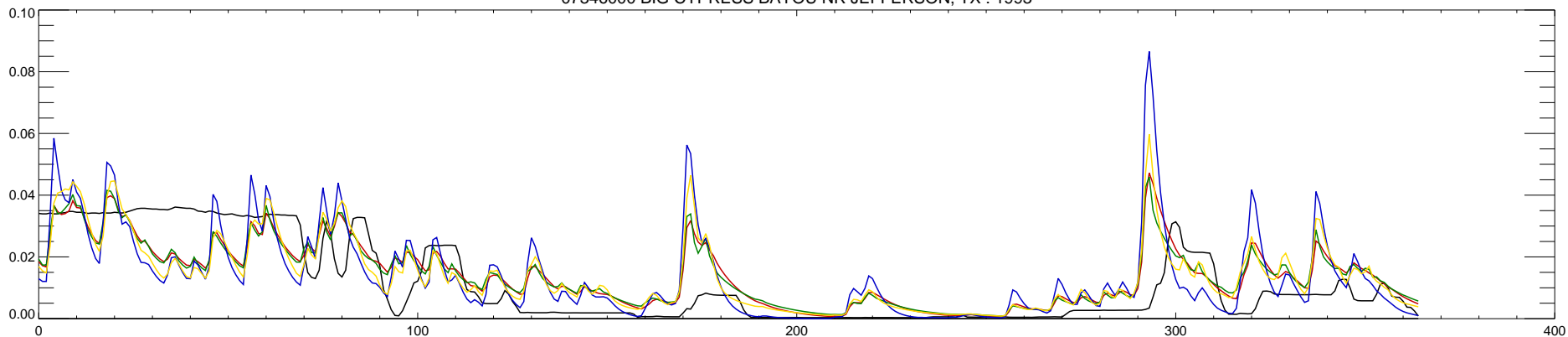
07346000 BIG CYPRESS BAYOU NR JEFFERSON, TX : 1994
