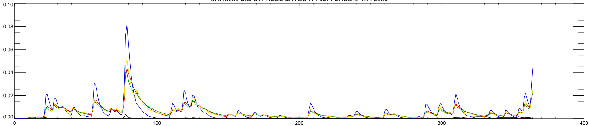
07346000 BIG CYPRESS BAYOU NR JEFFERSON, TX : 2007
