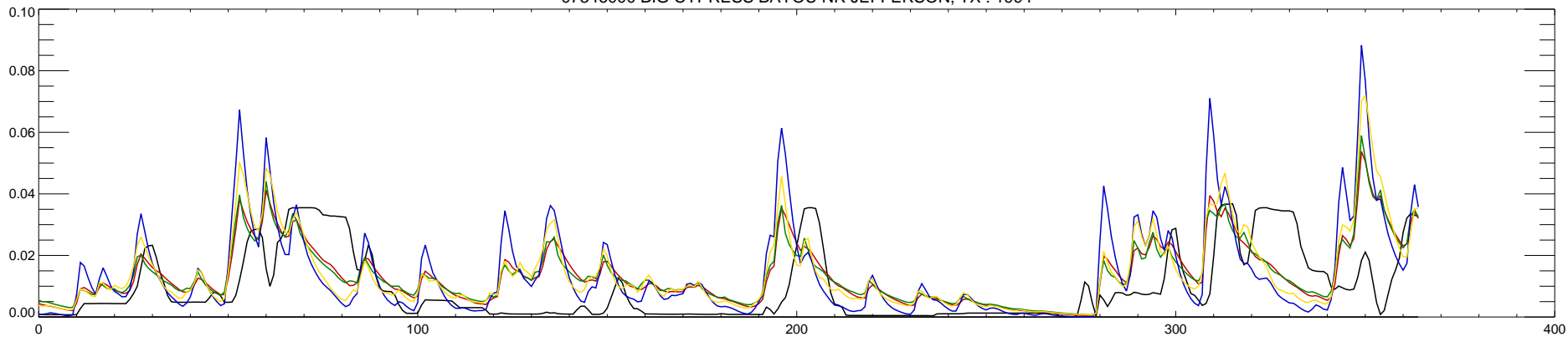
07346000 BIG CYPRESS BAYOU NR JEFFERSON, TX : 1995
