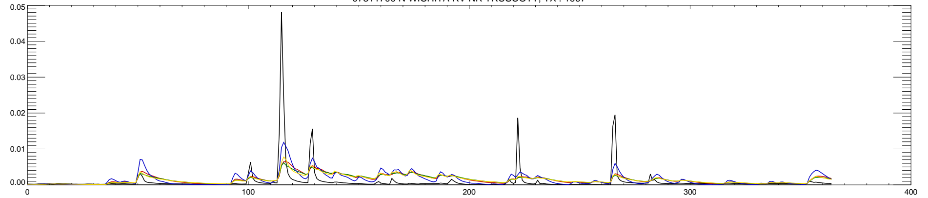
07311700 N WICHITA RV NR TRUSCOTT, TX : 1998
