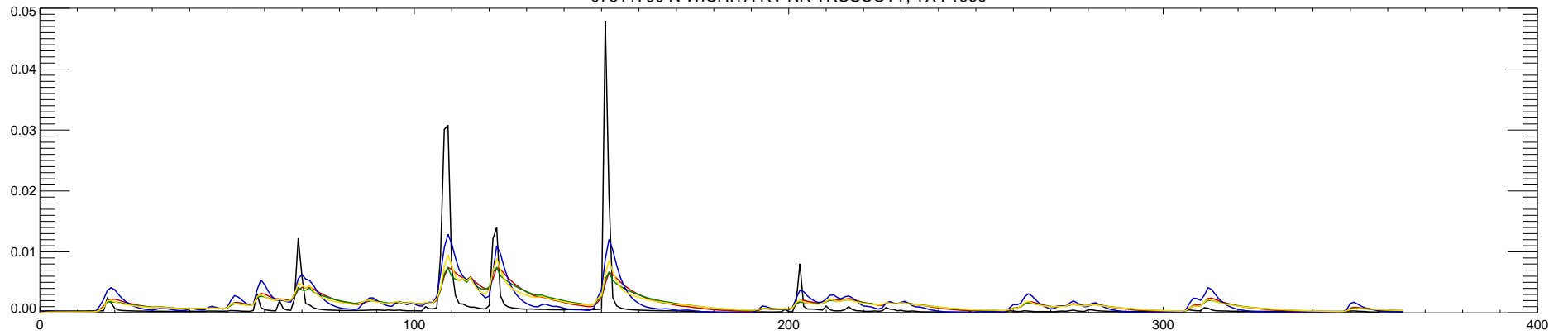
07311700 N WICHITA RV NR TRUSCOTT, TX : 1991
