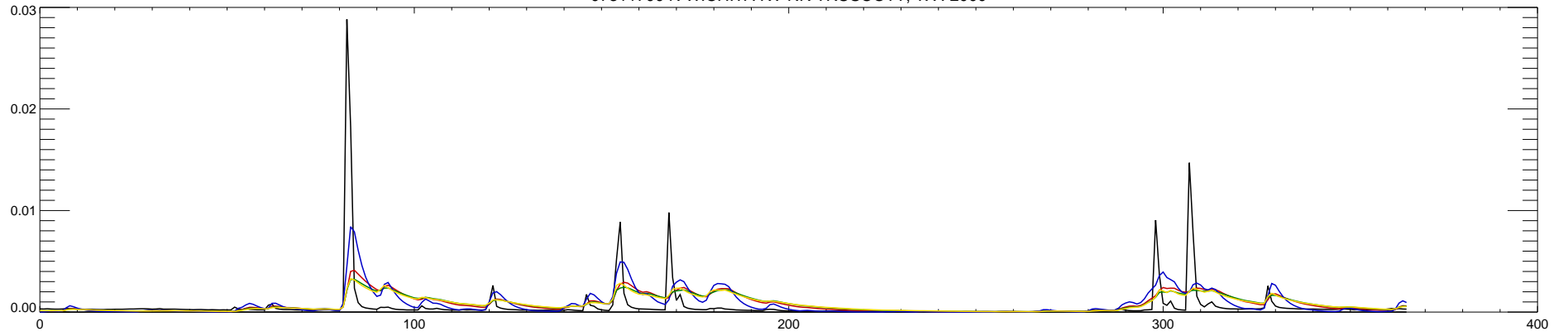
07311700 N WICHITA RV NR TRUSCOTT, TX : 2001
