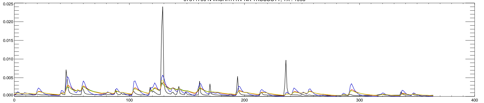
07311700 N WICHITA RV NR TRUSCOTT, TX : 1994
