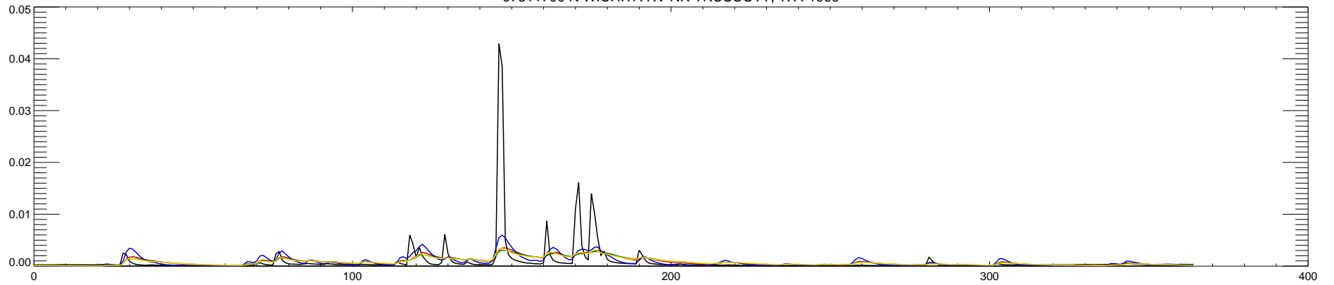
07311700 N WICHITA RV NR TRUSCOTT, TX : 2000
