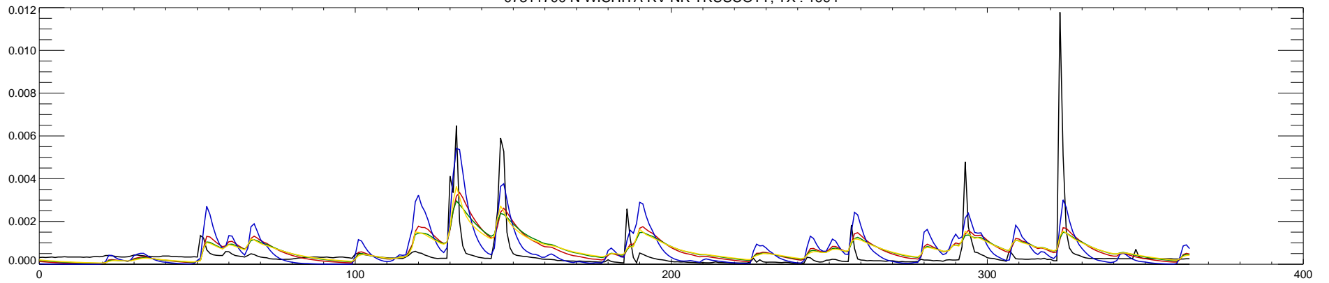
07311700 N WICHITA RV NR TRUSCOTT, TX : 1995
