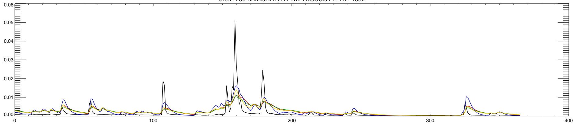
07311700 N WICHITA RV NR TRUSCOTT, TX : 1992
