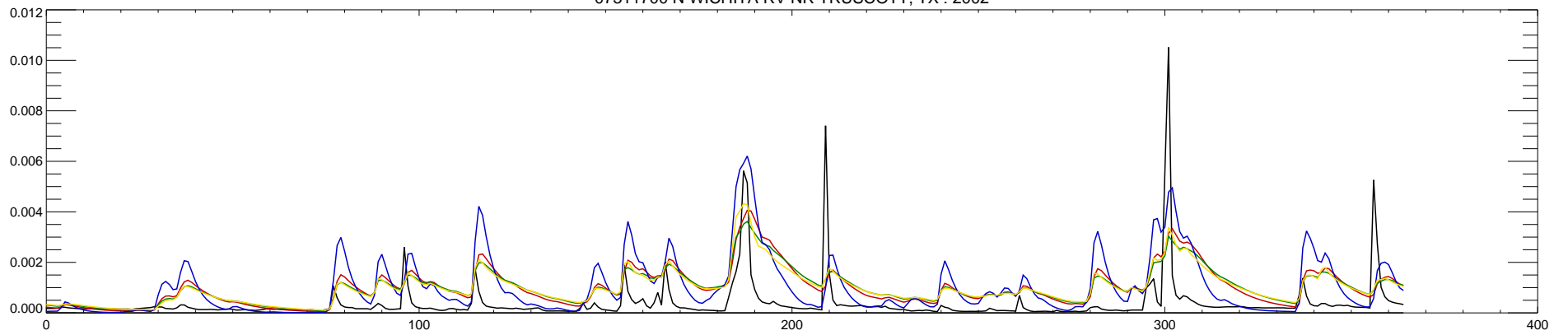
07311700 N WICHITA RV NR TRUSCOTT, TX : 2003
