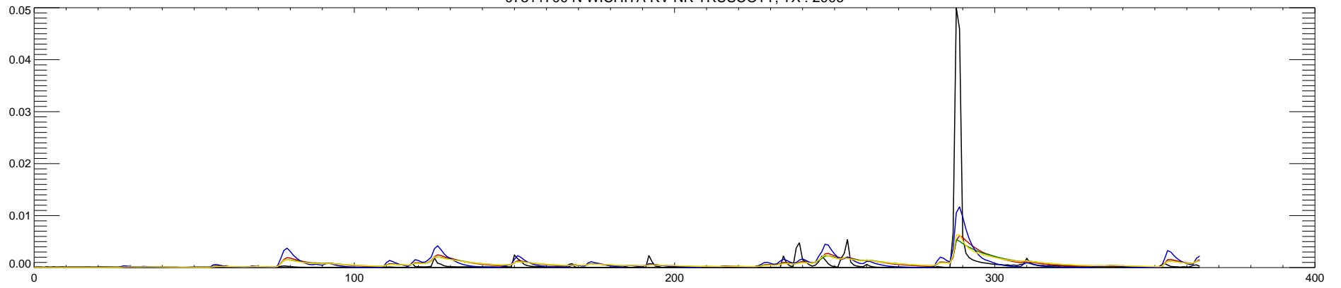
07311700 N WICHITA RV NR TRUSCOTT, TX : 2007
