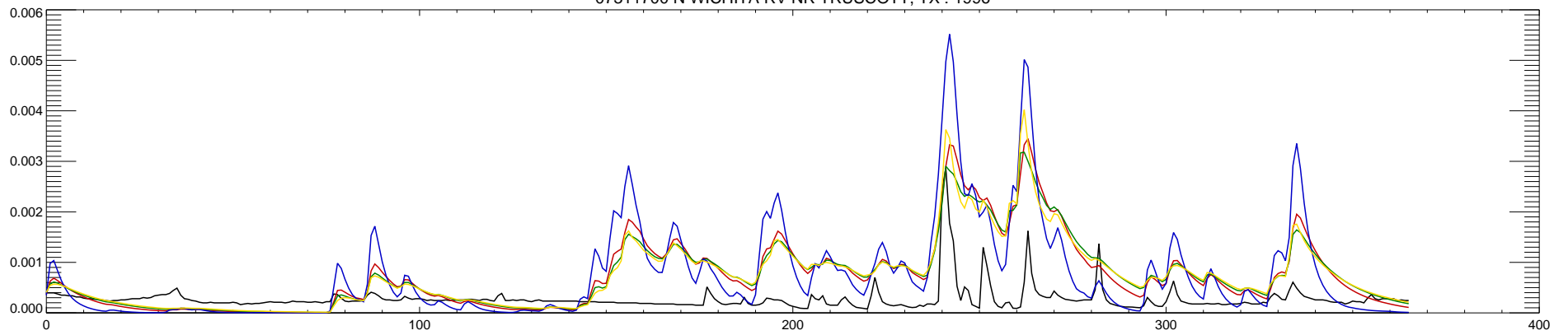
07311700 N WICHITA RV NR TRUSCOTT, TX : 1997
