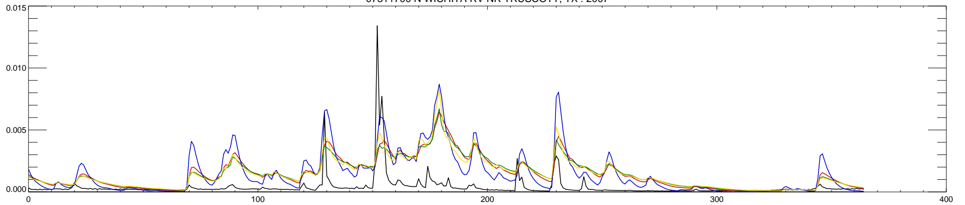
07311700 N WICHITA RV NR TRUSCOTT, TX : 2007
