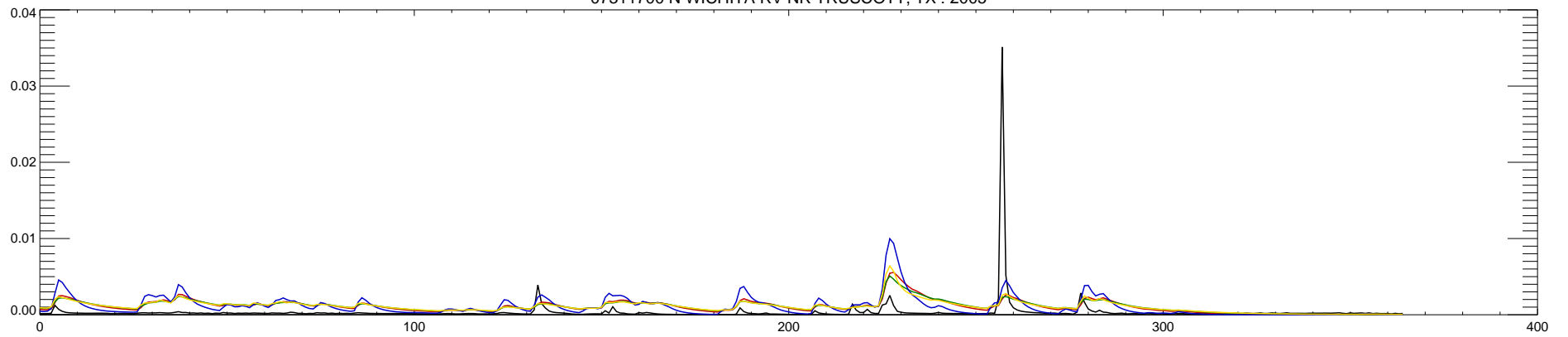
07311700 N WICHITA RV NR TRUSCOTT, TX : 2006
