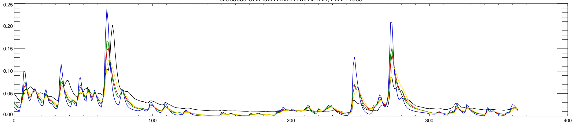
02359000 CHIPOLA RIVER NR ALTHA, FLA. : 1998
