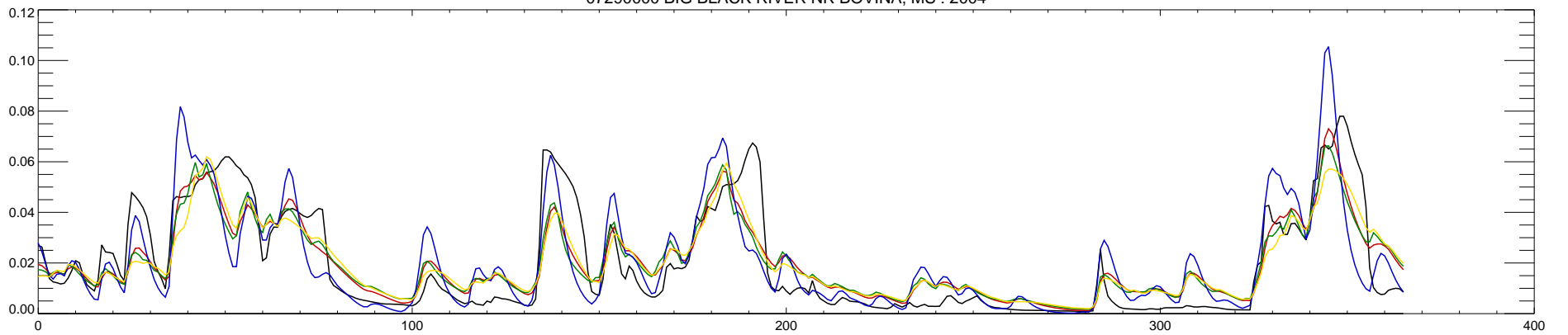
07290000 BIG BLACK RIVER NR BOVINA, MS : 2004
