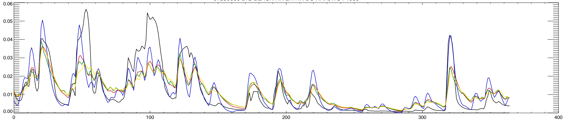
07290000 BIG BLACK RIVER NR BOVINA, MS : 1994
