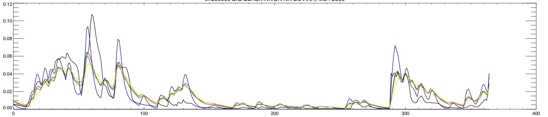
07290000 BIG BLACK RIVER NR BOVINA, MS : 2007
