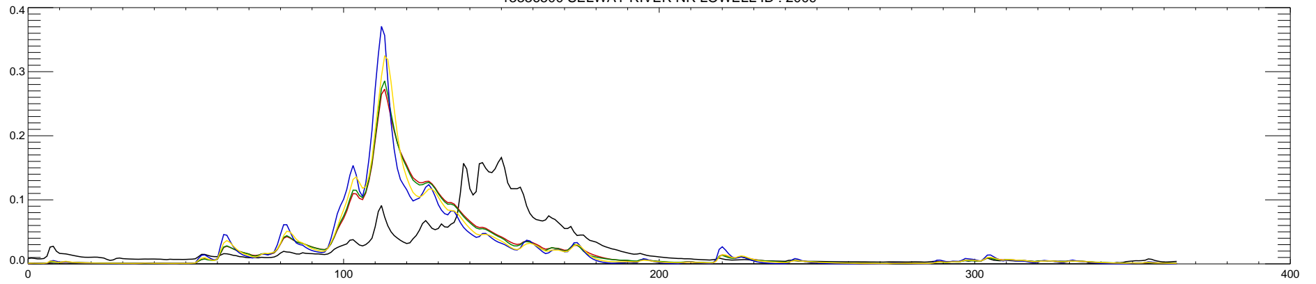
13336500 SELWAY RIVER NR LOWELL ID : 2009
