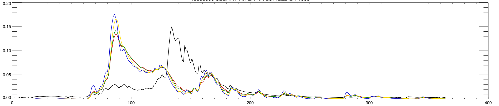
13336500 SELWAY RIVER NR LOWELL ID : 1994
