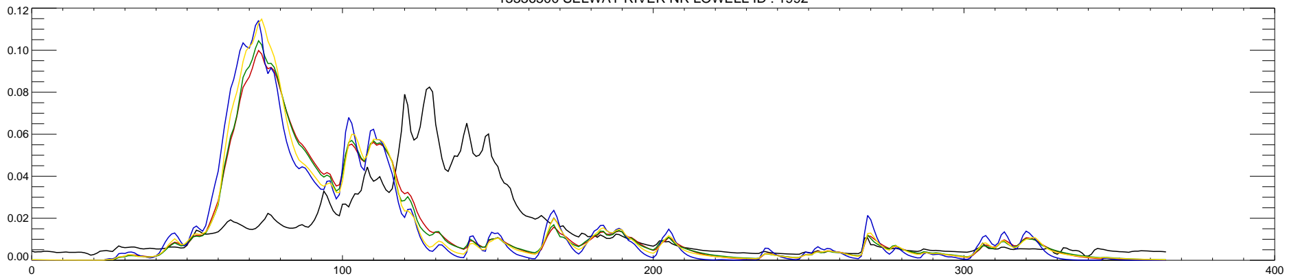
13336500 SELWAY RIVER NR LOWELL ID : 1992
