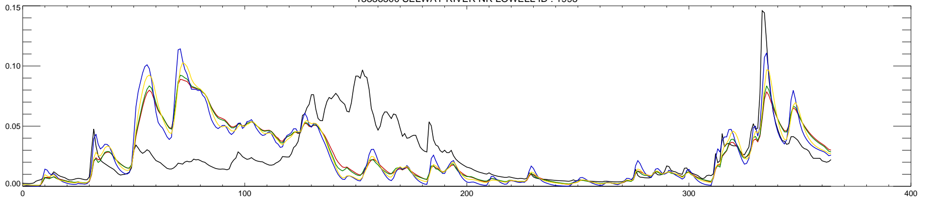
13336500 SELWAY RIVER NR LOWELL ID : 1995
