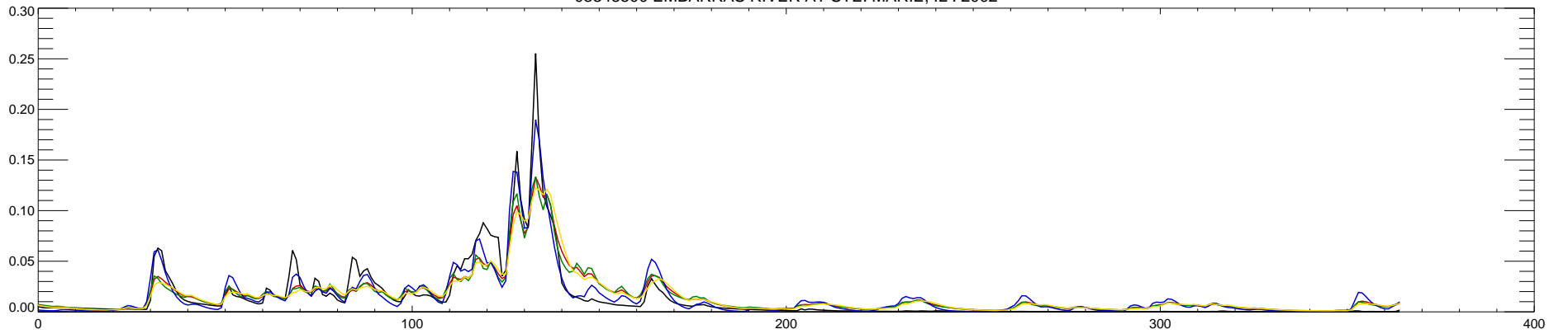
03345500 EMBARRAS RIVER AT STE. MARIE, IL : 2003
